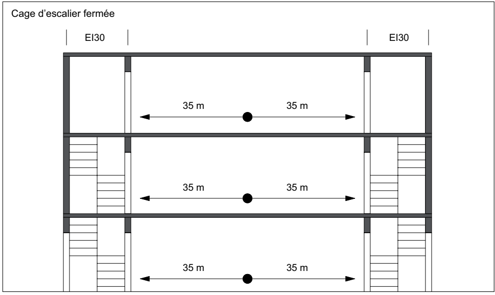
Longueur d'une voie d'évacuation dans les cas de plusieurs cages d'escaliers fermées (EI30)
